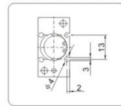
磁性开关安装槽位置
